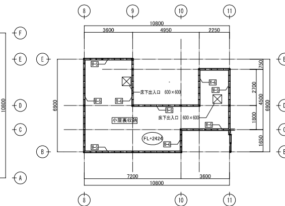
小屋裏平面図
