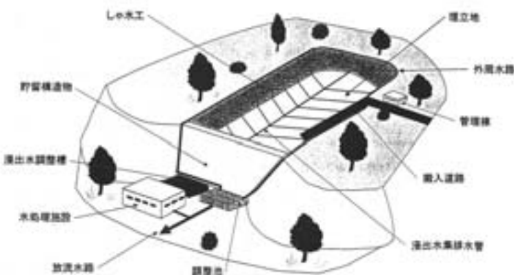
一般廃棄物最終処分場概念図
