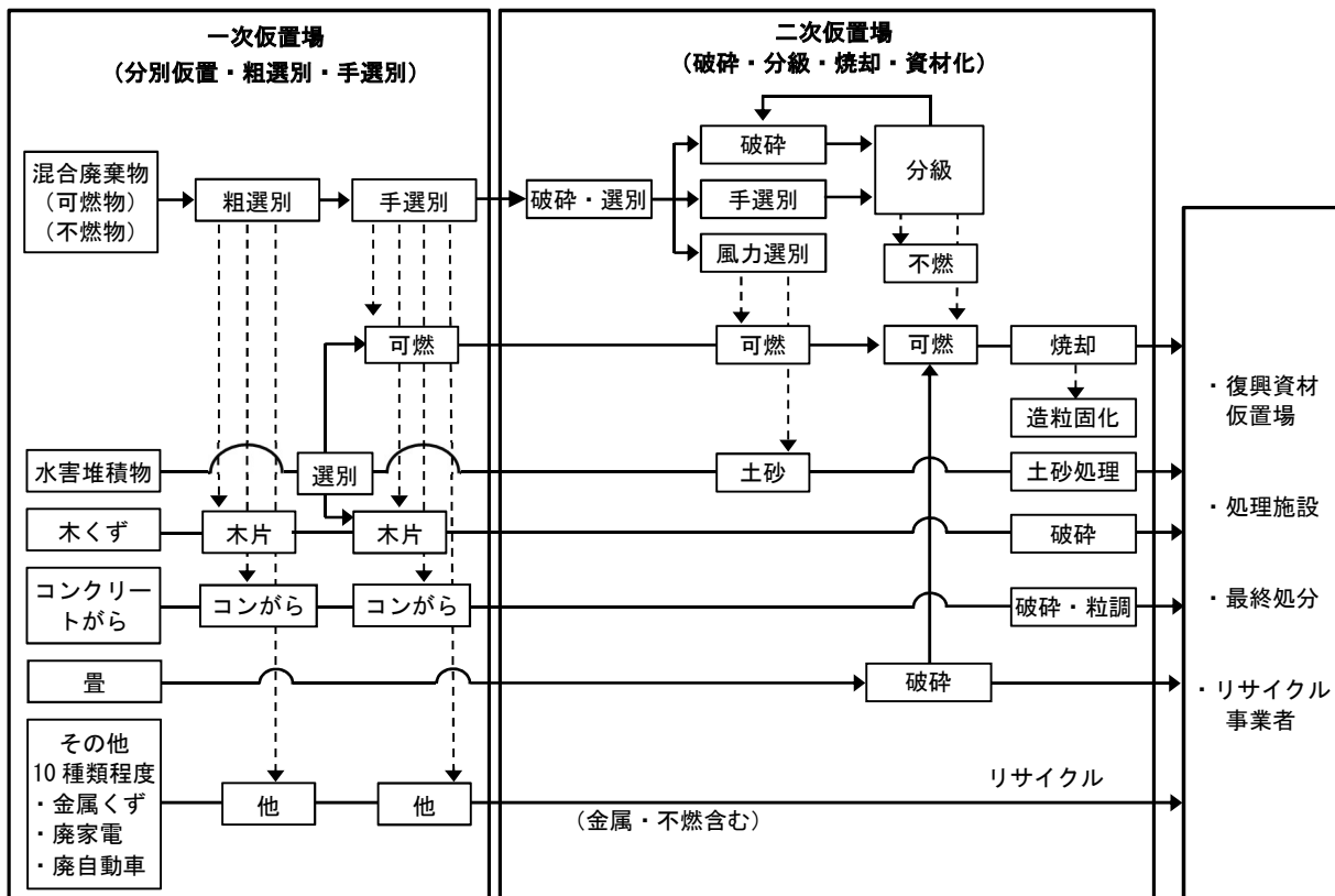
図表 2-2-10 災害廃棄物の基本的な処理フロー
