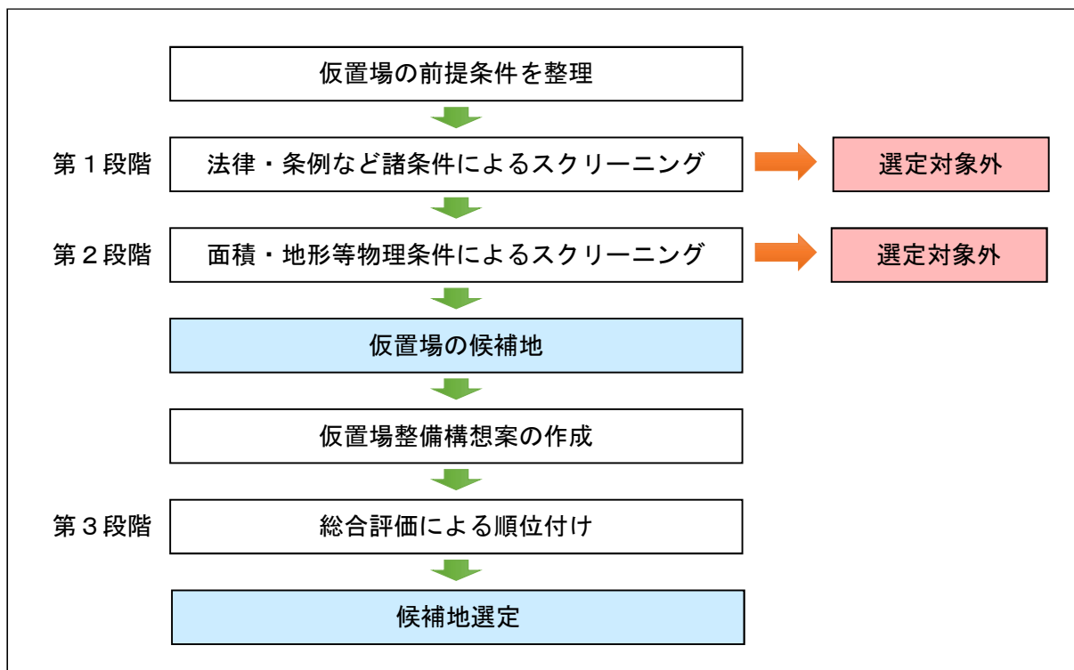
図表 2-2-13 仮置場の選定フロー
