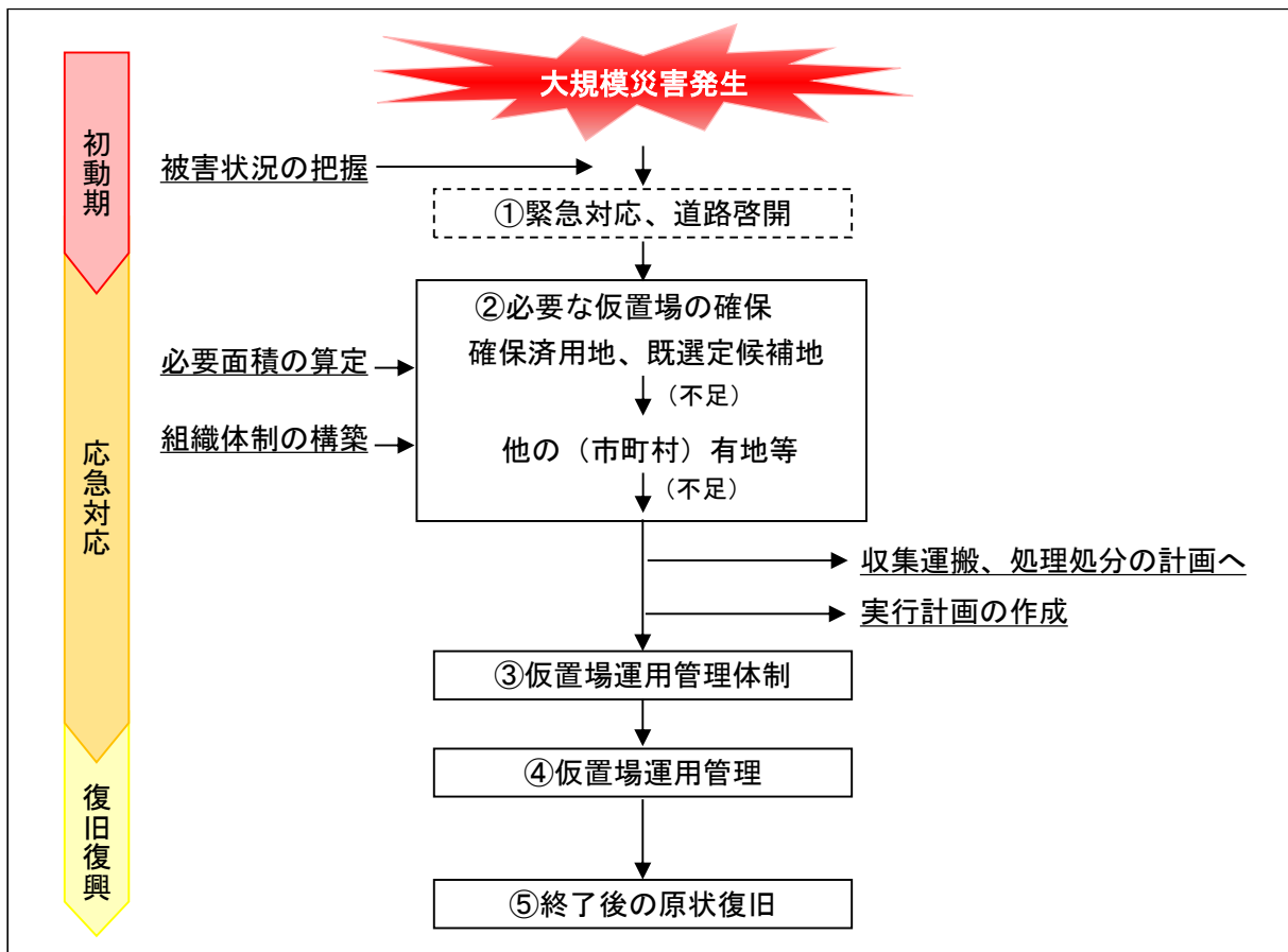
図表 3-2-6 仮置場の確保及び運営管理に係る対応フロー
